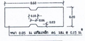
รูปขยาย ② 1:10
