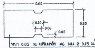
รูปขยาย ① 1:10
