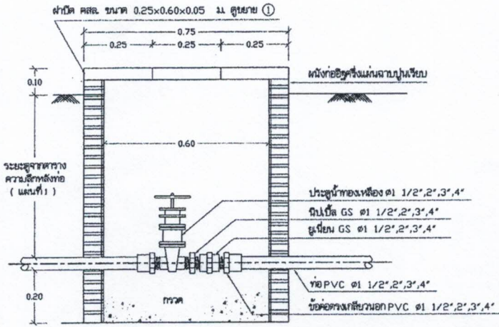
10. แบบการติดตั้งประตูปะบายอากาศอัตโนมัติ Ø 1 1/2", 2", 3", 4" 1:10
