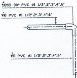
7. แบบการต่อข้อโค้ง 90° PVC
